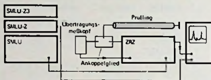
Bild 3. Resonanzmessung im Wobbelbetrieb mit Leistungs-Meßsender SMLU, Wobbelzusatz SMLU-Z, Frequenzkontrolller SMLU-Z3 und Reflexionsmesser ZRZ
