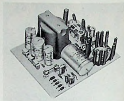
Bild 6. 180-W-Thyristorschaltnetzteil mit Netztrennung von Siemens
