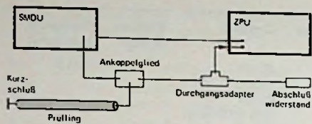
Bild 2. Meßaufbau für Dämpfungsmessungen nach dem Resonanzverfahren für manuellen Betrieb mit Universal-Meßsender SMDU und Vektorvollmeter ZPU
