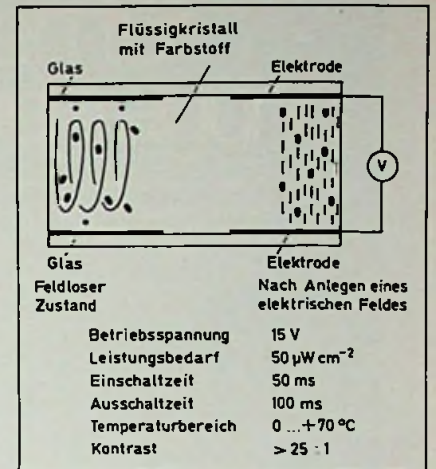
Bild 5. Aufbau und charakteristische Daten einer Flüssigkristallanzeige mit Bistabilitätseffekt
