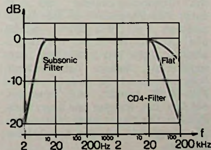
Bild 3. Übertragungsbereich und Frequenzgang U_a = f(f) des Vorverstärkers MCA 76
