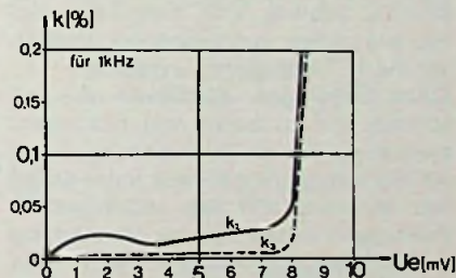
Bild 2. Der quadratische ( k_2 ) und der kubische ( k_3 ) Klirrgrad des Verstärkers MCA 76 in Abhängigkeit von der Eingangsspannung U_e .
