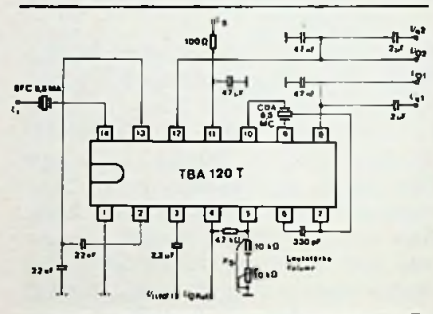
Bild 3. TBA 120 T von AEG-Telefunken bei Verwendung von Keramik-Resonatoren
